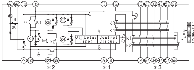
G9SA-TH301型 (AC/DC24V)
