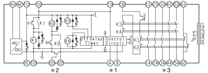
G9SA-TH301型 (AC100~240V)
