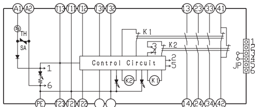
G9SA-TH301型 (AC/DC24V)
