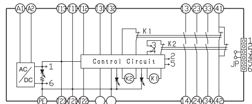
G9SA-TH301型 (AC100~240V)
