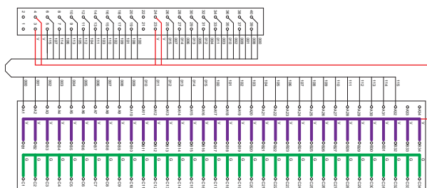
XW2K-40G-O32C-IN
