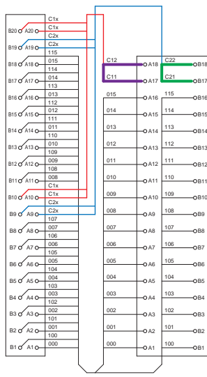
XW2K-40G-032B
