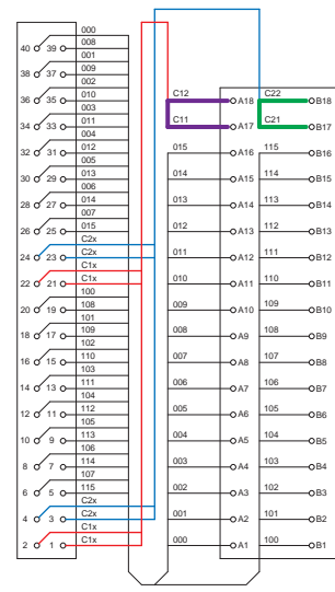
XW2K-40G-032C
