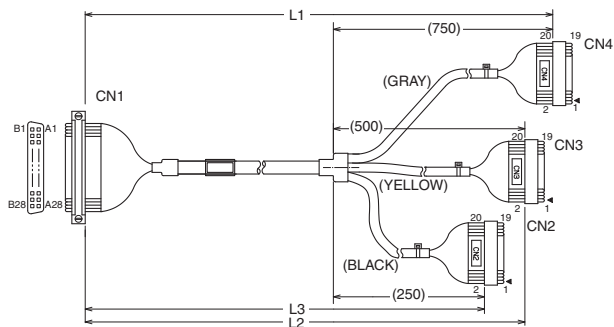
CN4 : XG4M-2030-T
